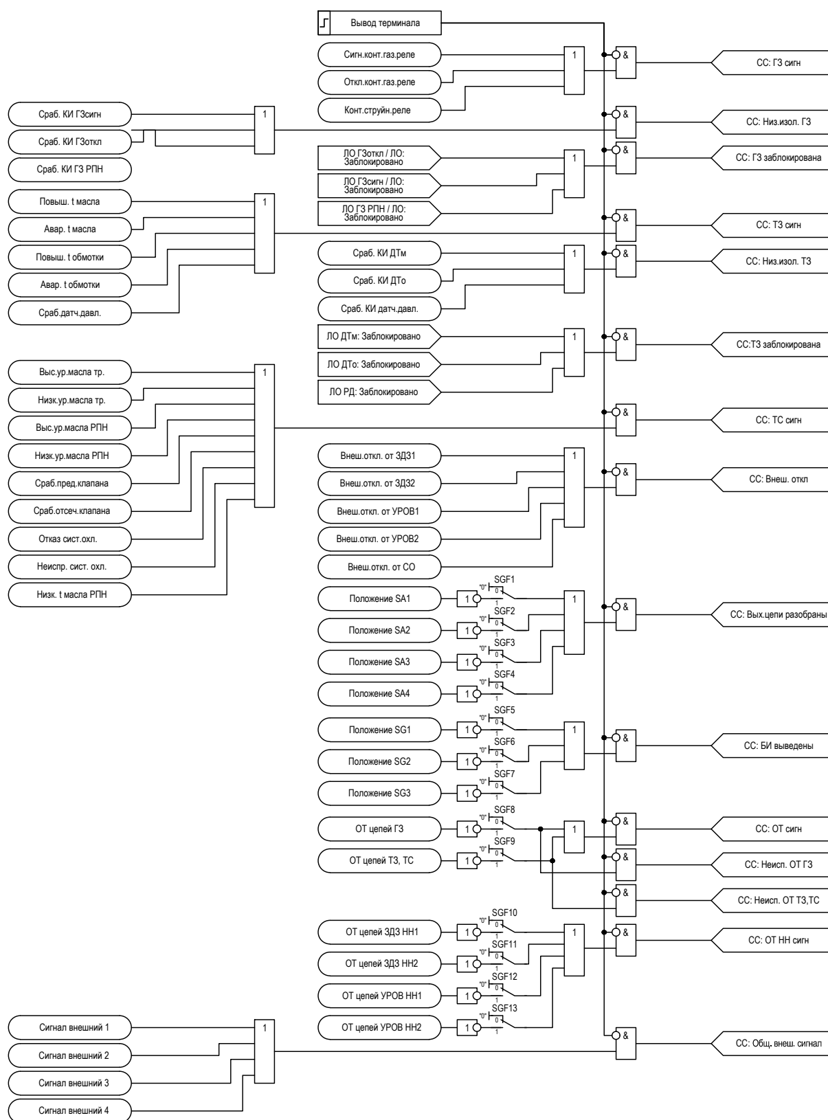
Рисунок 2.32 – Функциональная схема логики сборки сигналов
